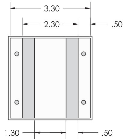
仰视图
