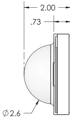
侧视图
